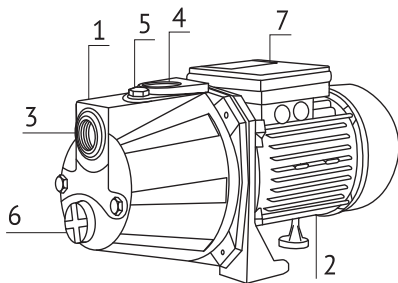
Рисунок 5. Центробежный насос серии JET-S.
