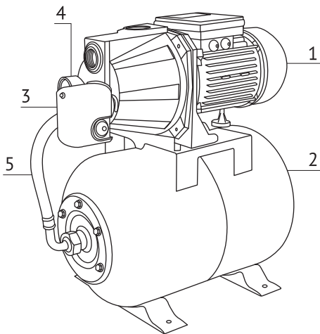
Рисунок 6. Насосная станция на базе центробежного насоса серии JET-S.
