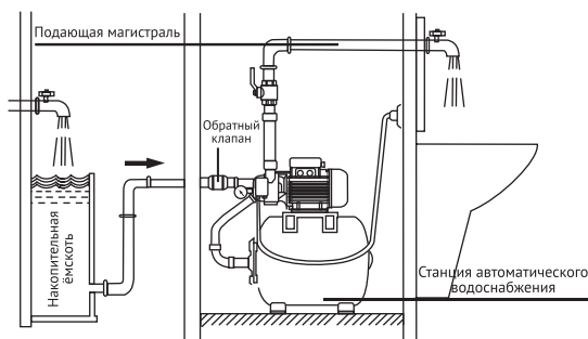
Рисунок 3. Система водоснабжения из магистрального трубопровода через промежуточную накопительную емкость с использованием насосной станции на базе центробежного насоса JET-S.
