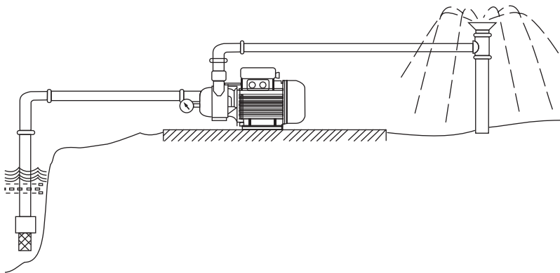
Рисунок 1. Система полива без автоматического управления работой насоса.
