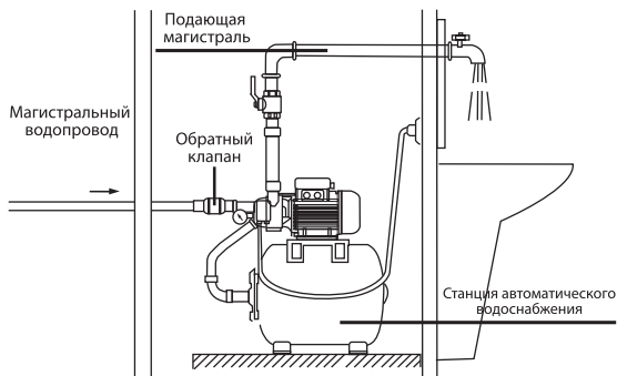
Рисунок 4. Система водоснабжения из магистрального трубопровода без промежуточной накопительной емкости с использованием насосной станции на базе центробежного насоса JET-S.
