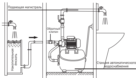
Рисунок 3. Система водоснабжения из магистрального трубопровода через промежуточную накопительную емкость с использованием насосной станции на базе центробежного насоса JET-P.
