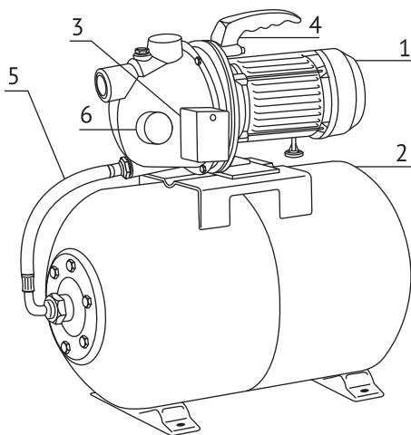
Рисунок 6. Насосная станция на базе центробежного насоса серии JET-P.
