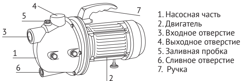
Рисунок 5. Центробежный насос серии JET-P.
