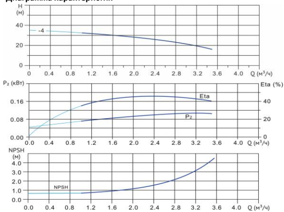
Диаграмма характеристик
