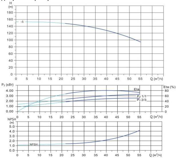
Диаграмма характеристик
