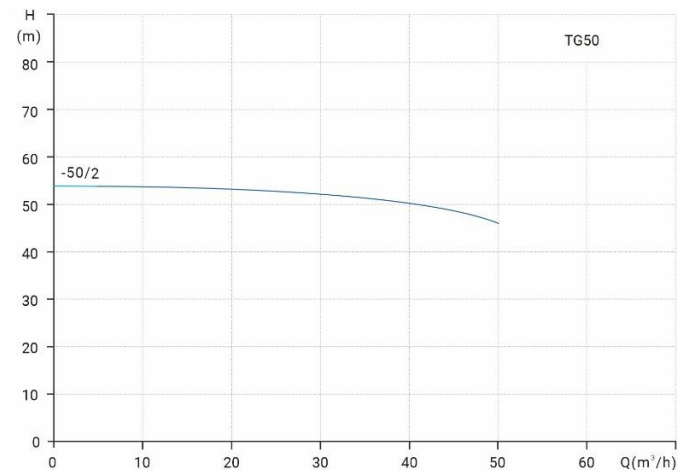
Диаграмма характеристик
