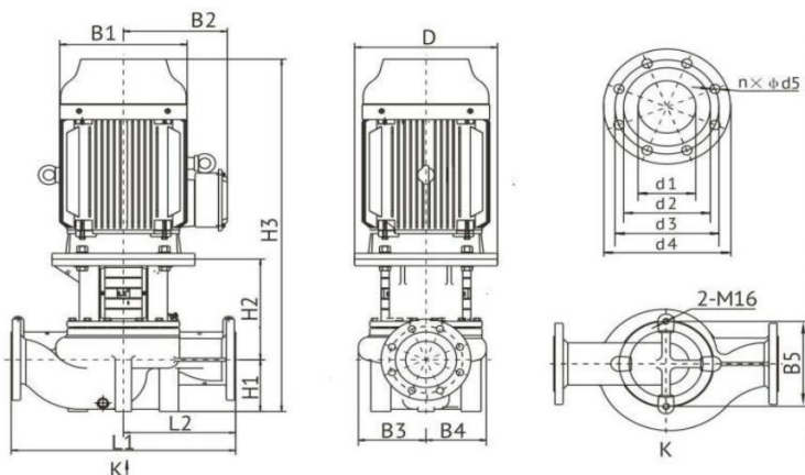
Габаритный чертёж
