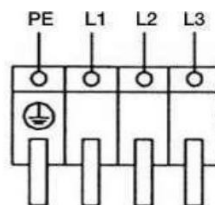
Схема электроподключения
