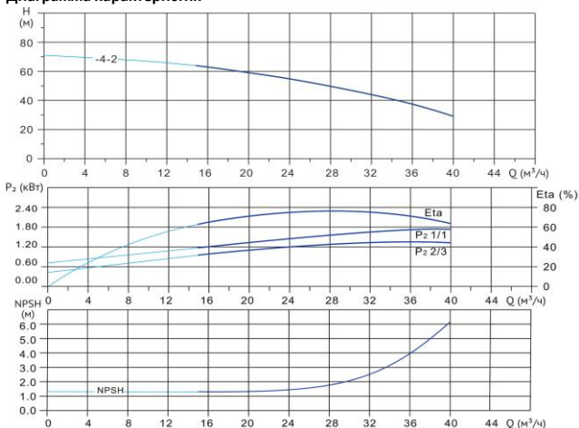
Диаграмма характеристик
