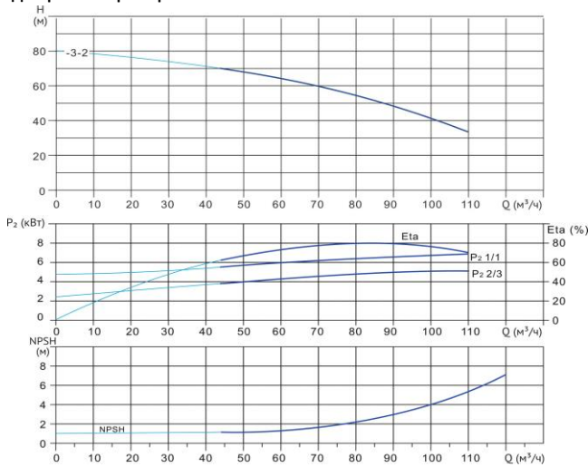
Диаграмма характеристик
