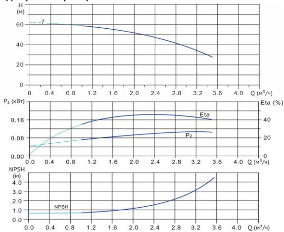
Диаграмма характеристик
