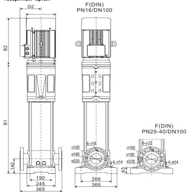
Размеры, мм
