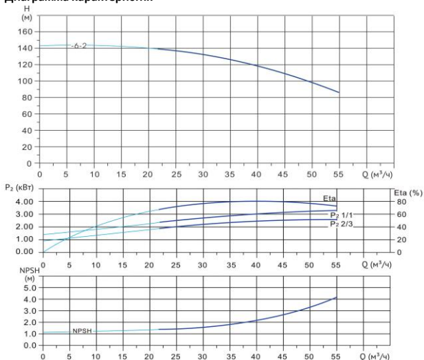
Диаграмма характеристик
