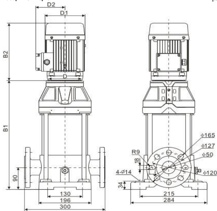
Размеры, мм
