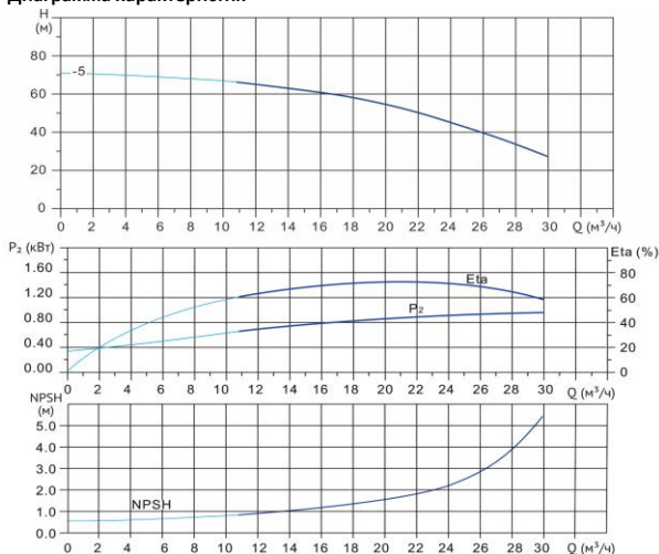
Диаграмма характеристик
