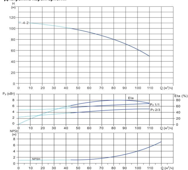
Диаграмма характеристик
