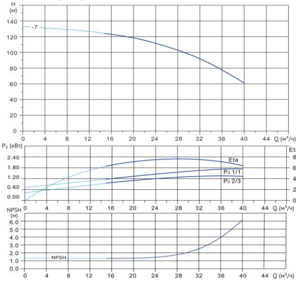
Диаграмма характеристик
