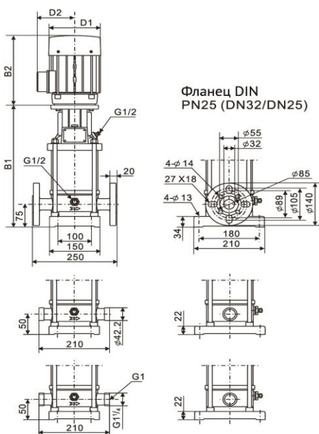
Размеры, мм
