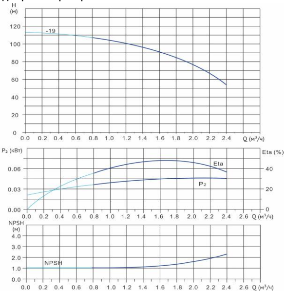
Диаграмма характеристик
