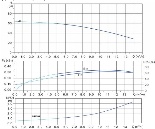
Диаграмма характеристик
