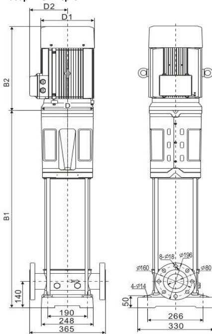
Размеры, мм
