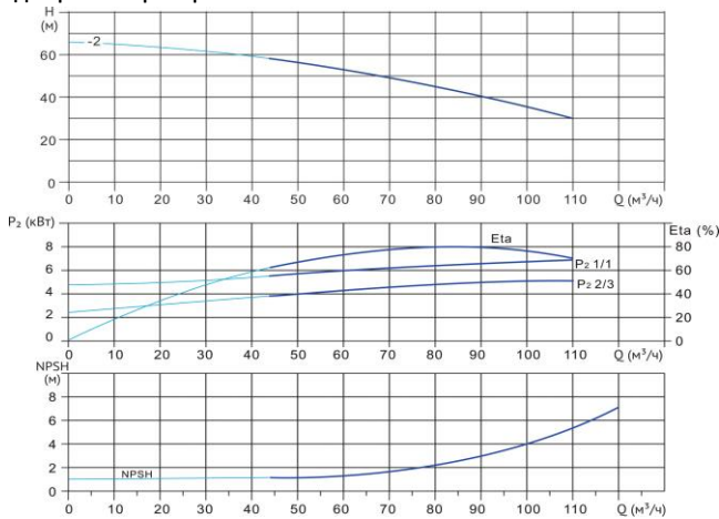
Диаграмма характеристик
