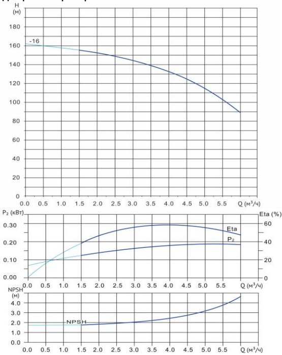
Диаграмма характеристик
