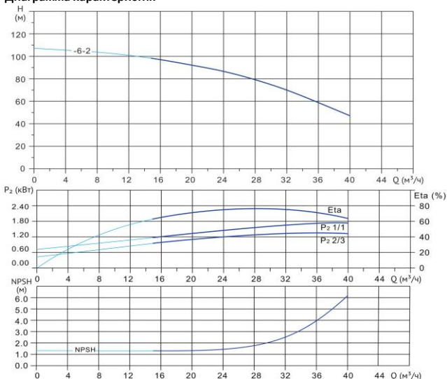
Диаграмма характеристик
