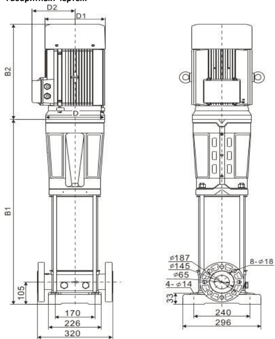
Размеры, мм
