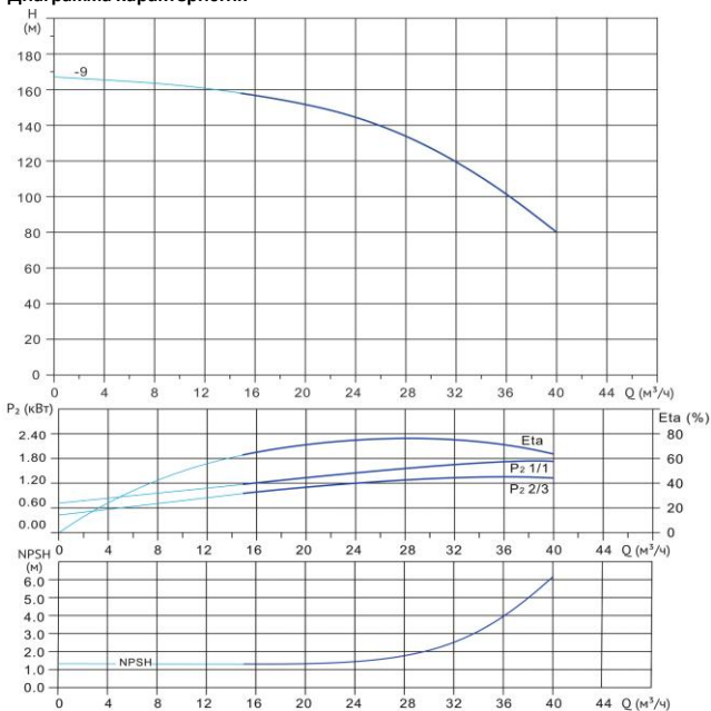
Диаграмма характеристик
