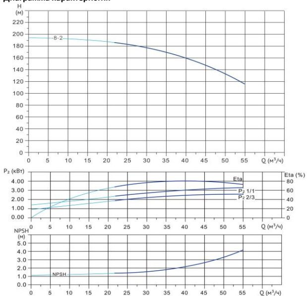
Диаграмма характеристик
