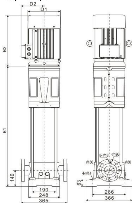
Размеры, мм
