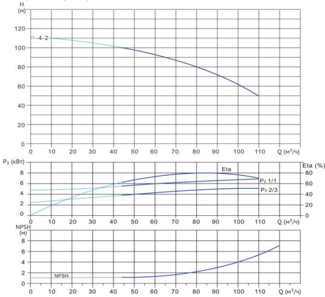
Диаграмма характеристик
