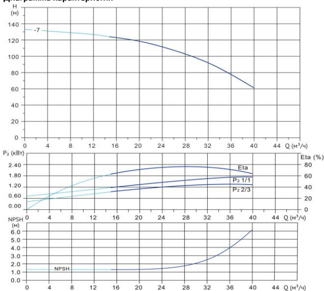
Диаграмма характеристик
