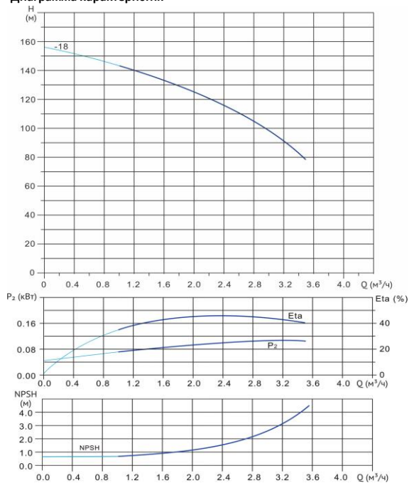
Диаграмма характеристик
