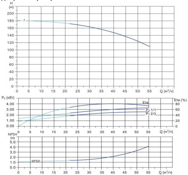
Диаграмма характеристик
