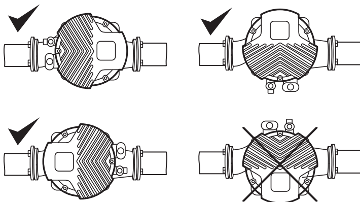
Рисунок 3. Допустимые положения блока управления отмечено ✓
