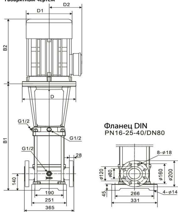
Размеры, мм
