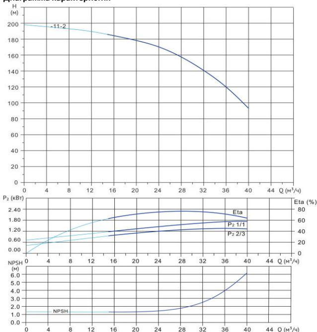
Диаграмма характеристик
