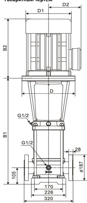
Размеры, мм
