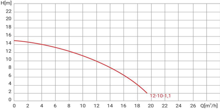
Диаграмма характеристик
