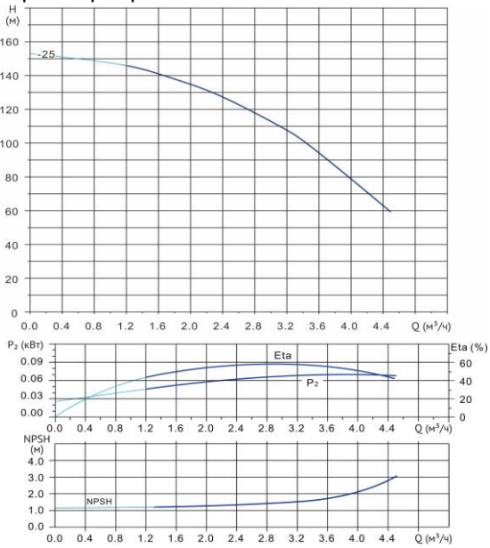
Диаграмма характеристик
