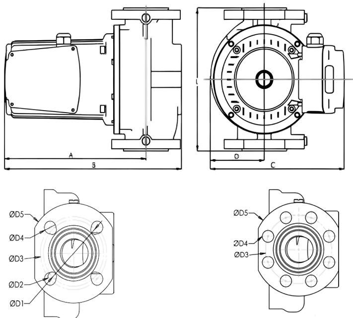
Размеры фланца 80
