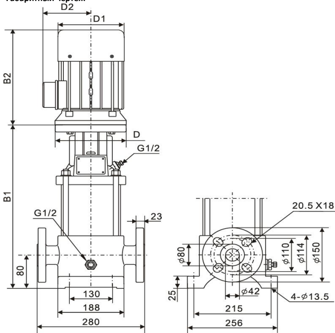
Габаритный чертёж
