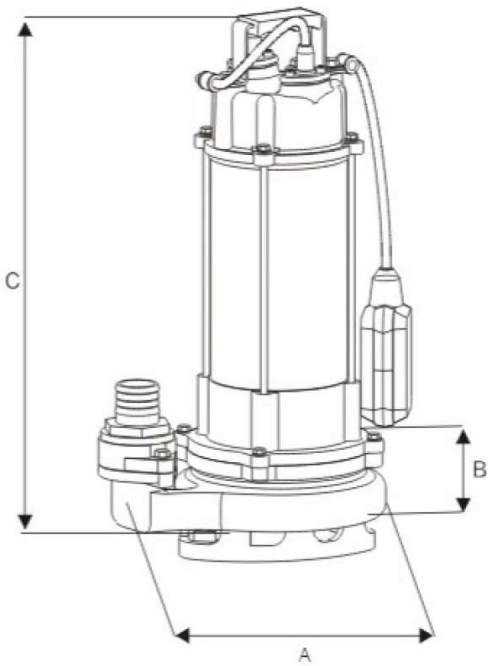
Габаритные размеры
