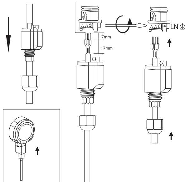
Рисунок 5. Электрическое подключение
