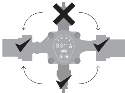
Рисунок 3. Допустимые положения блока управления
