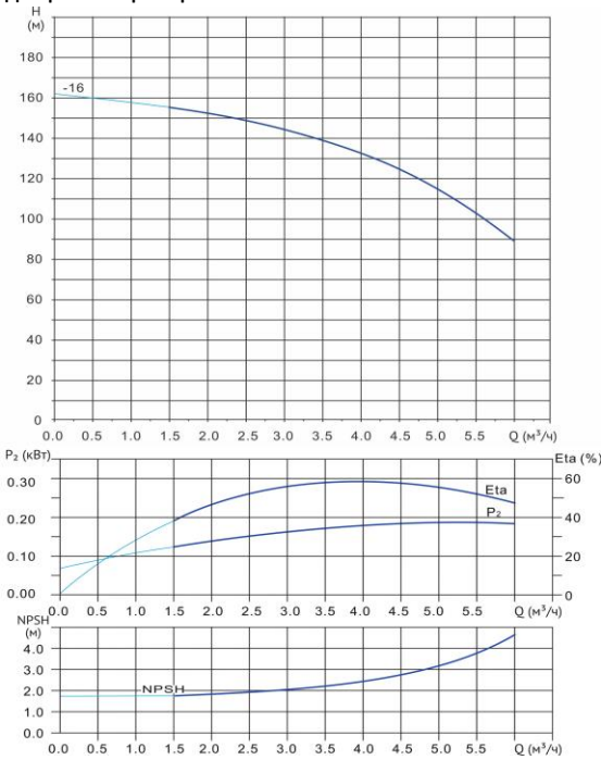
Диаграмма характеристик
