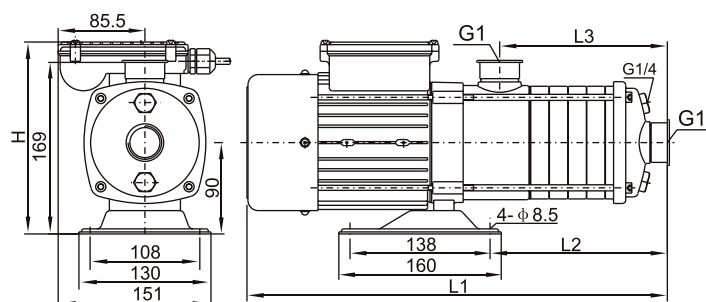
Габаритный чертеж
