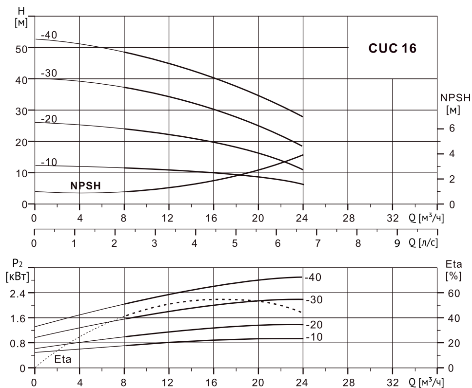
Диаграмма характеристик
