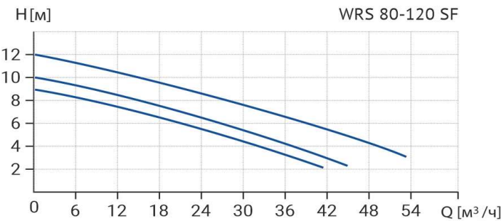
Диаграмма характеристик
