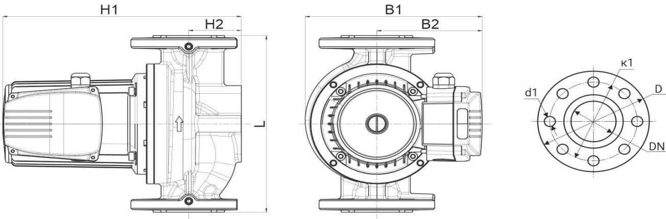
Габаритный чертёж
