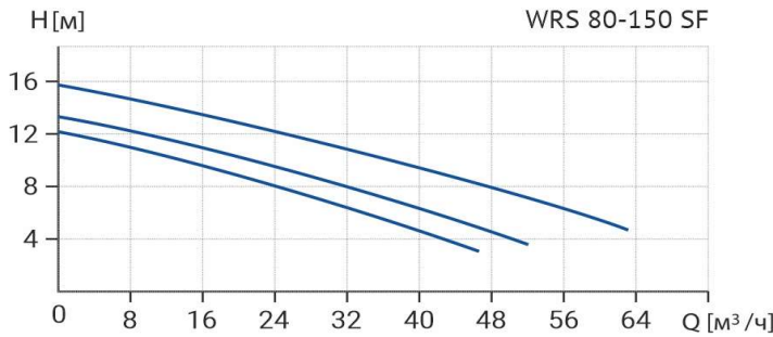
Диаграмма характеристик
