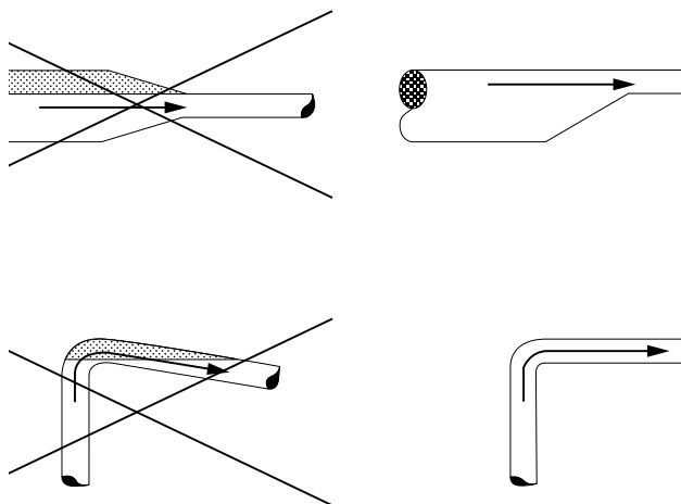
Рисунок 6. Конфигурация трубопроводов на всасывающей стороне.
