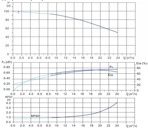
Диаграмма характеристик
