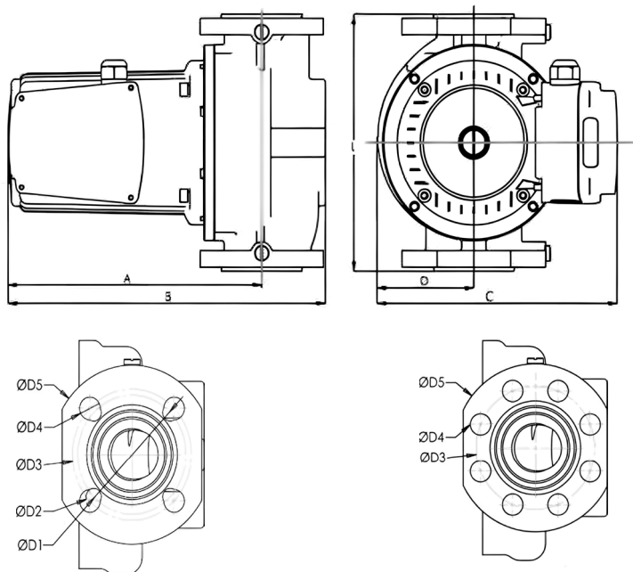
Размеры фланца 80
