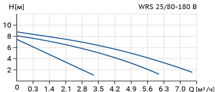
Диаграмма характеристик
