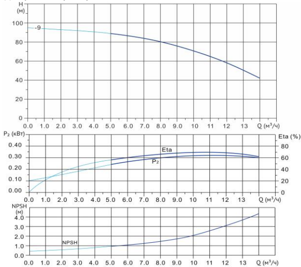
Диаграмма характеристик
