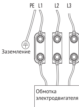
Рисунок 2. Схема электрического подключения
