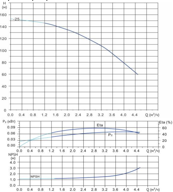
Диаграмма характеристик
