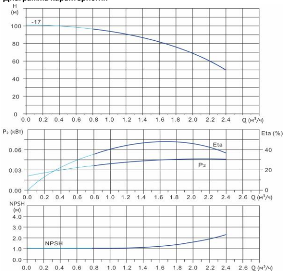
Диаграмма характеристик
