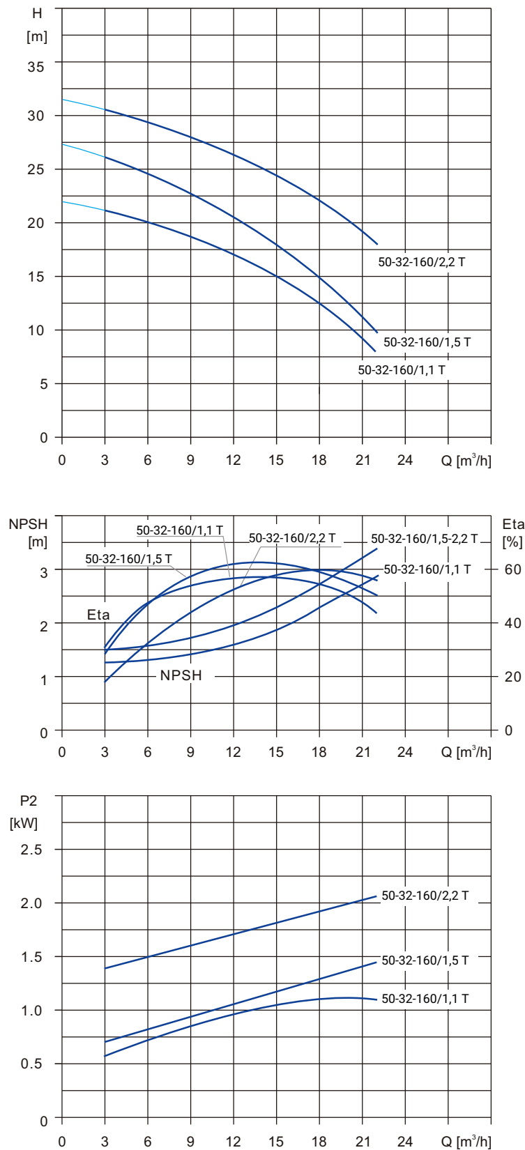
Рис.1. Пример графиков напор-расход, мощность, КПД, NPSH
