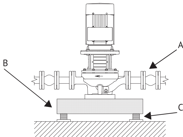
Рисунок 9. Способы устранения шума и вибраций.
