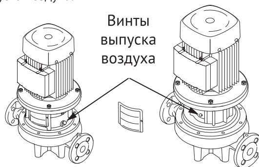
Рисунок 12. Вент выпуска воздуха.
