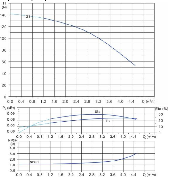
Диаграмма характеристик
